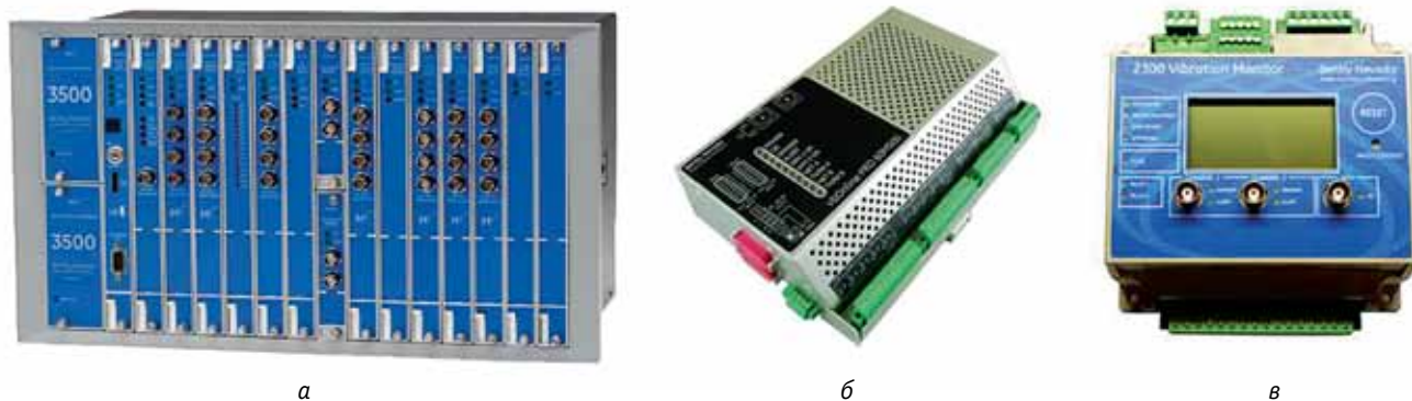
Рис. 3. Мониторы системы вибрационного мониторинга компании Bently Nevada: а – BN 3500; б – vbOnline Pro; в – BN 2300
