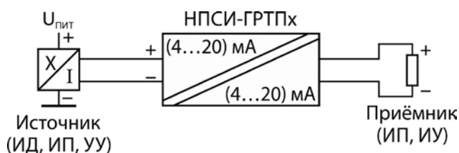
Рис. 3. Подключение преобразователей НПЦИ-ГРТП к активному источнику
