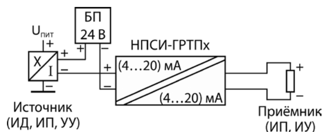
Рис. 4. Подключение преобразователей НПЦИ-ГРТП к пассивному источнику с применением дополнительного блока питания БП
