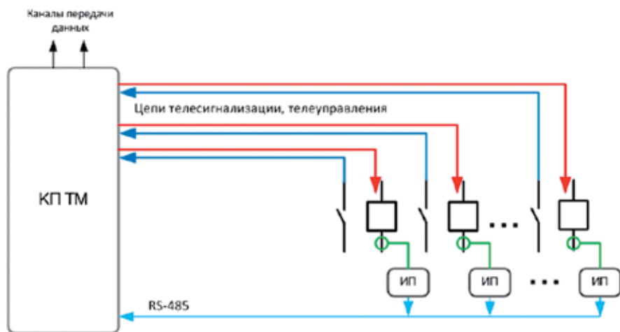
Рис. 2. Схема системы телемеханики со смешанной архитектурой
