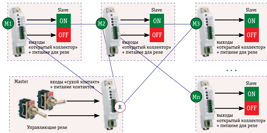
Рис. 5. Двухканальный адресный повторитель состояния контактов (Master → 1...32 Slave)
