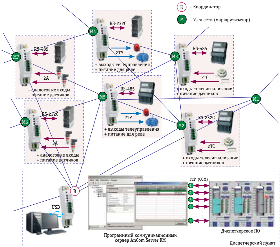
Рис. 2. Адресный доступ к объектам автоматизации со стороны диспетчерского ПО (ОС Windows)
