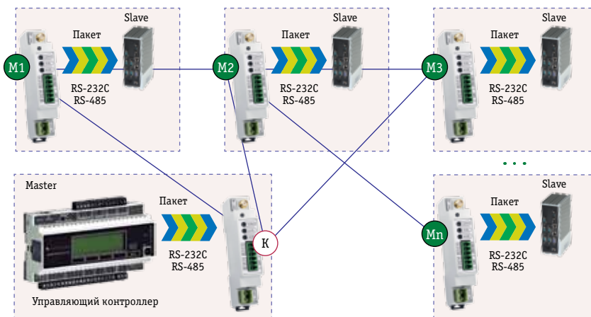
Рис. 4. Широковещательная ретрансляция данных из управляющего контроллера объектам автоматизации (неразрывные пакеты данных до 84 байт)
