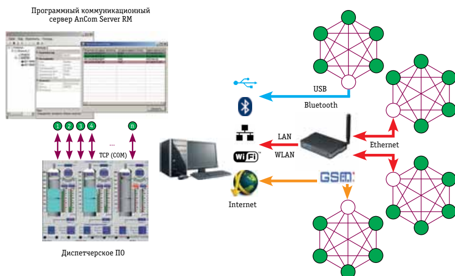
Рис. 6. Шлюз удаленного доступа в сеть ZigBee: подключение модема-координатора (пример для систем с адресным доступом к объектам автоматизации со стороны диспетчерского ПО Windows)
