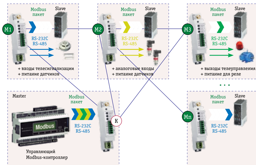
Рис. 3. Адресный доступ управляющего контроллера к объектам автоматизации по Modbus RTU (Master → 1...32 Slave, неразрывные пакеты данных до 255 байт)
