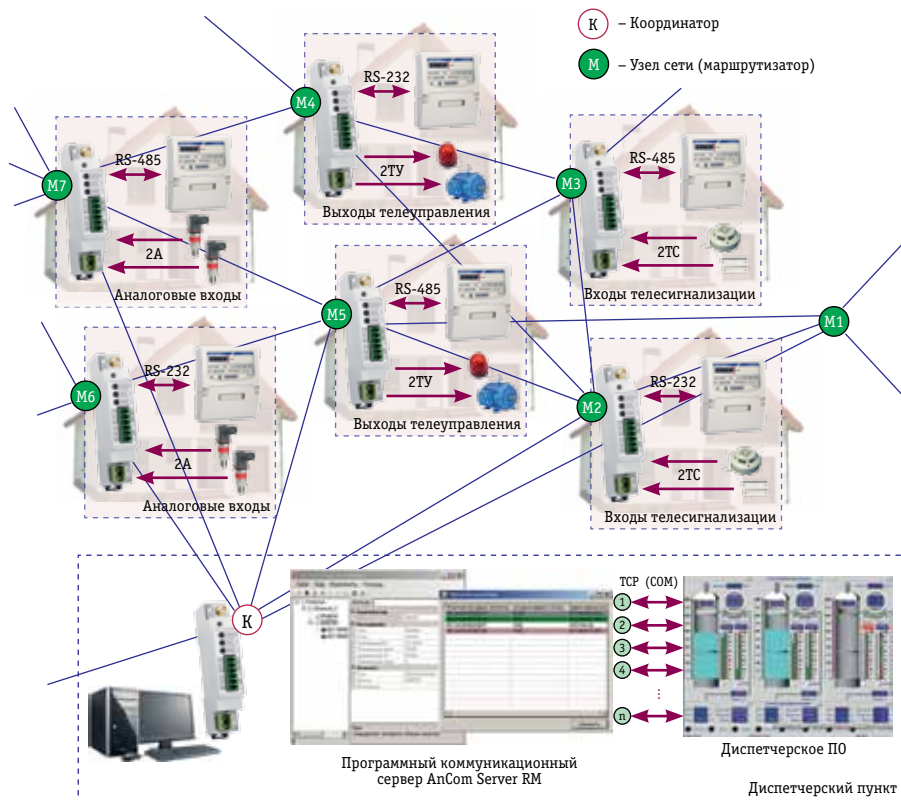
Рис. 2. Адресный доступ к приборам учета со стороны диспетчерского ПО (ОС Windows) и ретрансляция данных между маршрутизаторами (М) для связи с удаленным координатором (К)
