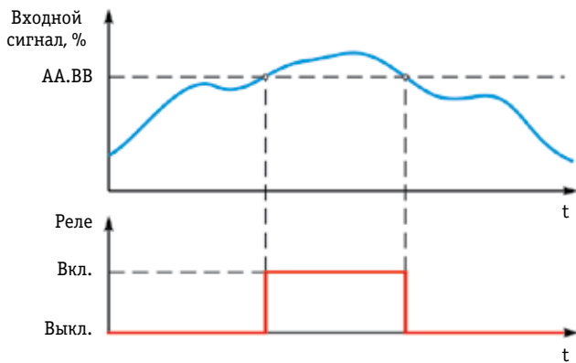
Рис. 2. Диаграмма работы сигнализации «превышение» без защелки
