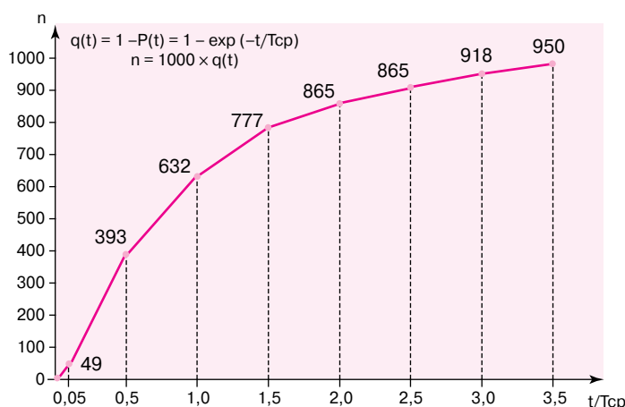
Рис. 1. Зависимость числа отказавших элементов от времени работы q(t) = 1 - P(t) = 1 - \exp(-t/T_{ср}) n = 1000 \times q(t)
