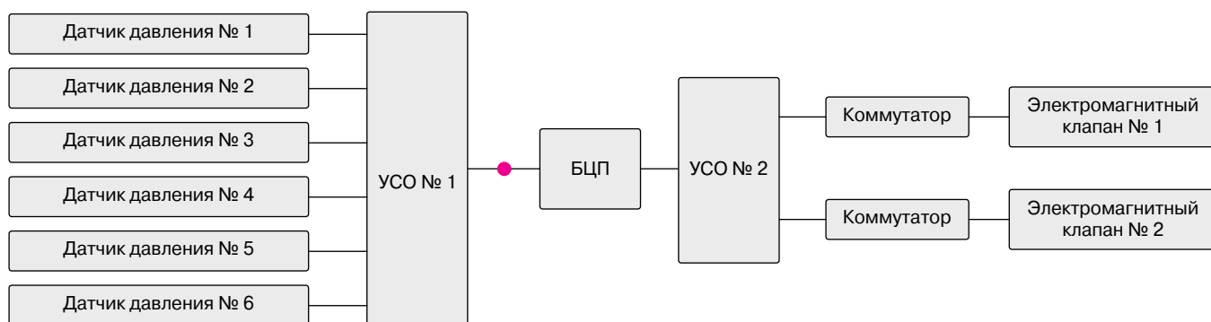
Рис. 2. Структура гипотетической системы защит котла
