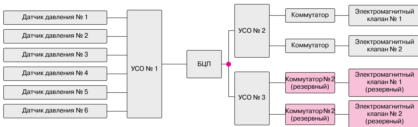
Рис. 3. Структурная схема гипотетической системы защиты котла с резервированием наиболее ненадежных элементов
