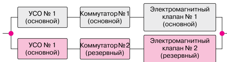
Рис. 4. Структурная схема резервированного узла для расчета надежности
