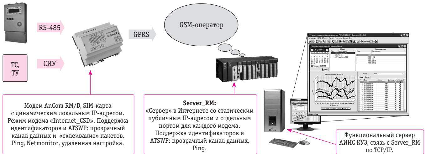
Рис.1. Схема АИИС КУЭ ППЭ, ООО «Волгаэнергоприбор», г. Самара
