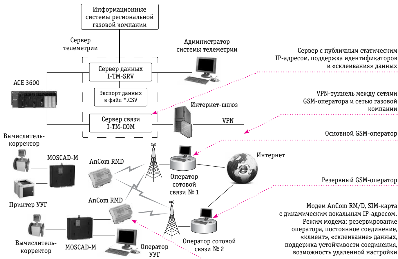
▲ Схема организации GPRS-канала системы «MOSCAD»
