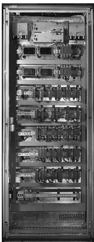
▲ Шкаф управления на базе контроллера ЭМИКОН
